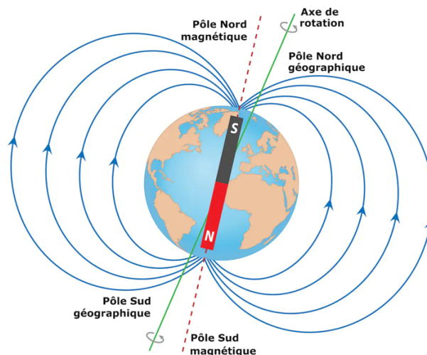
Le champ magnétique terrestre peut être vu comme celui d'un aimant droit légèrement décalé par rapport à l'axe de rotation de la Terre (pôle Nord géographique). Le Pôle Nord magnétique correspond en fait au pôle sud de l'aimant terrestre. OSweetNature/Shutterstock
